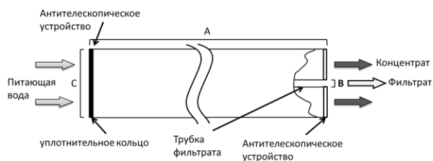
рис. 1а: схема размеров элемента со скрытой трубкой фильтра
